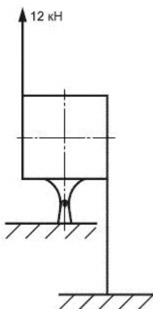
Рисунок 2 - Подвижное устройство
